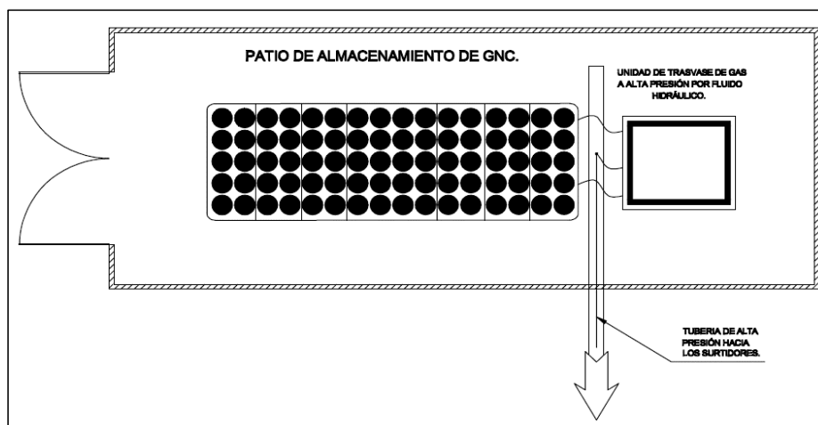
Figura 3 - Trasvase del GNC por medio de un fluido hidráulico
