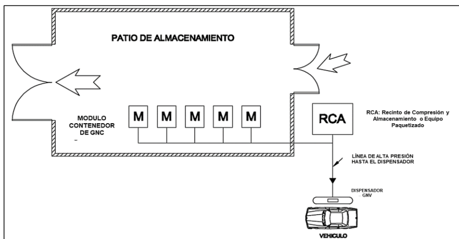
Figura 2B - Esquema referencial de una estación de descarga de GNC que descarga a una estación de GNV con pared divisoria 4TRF
