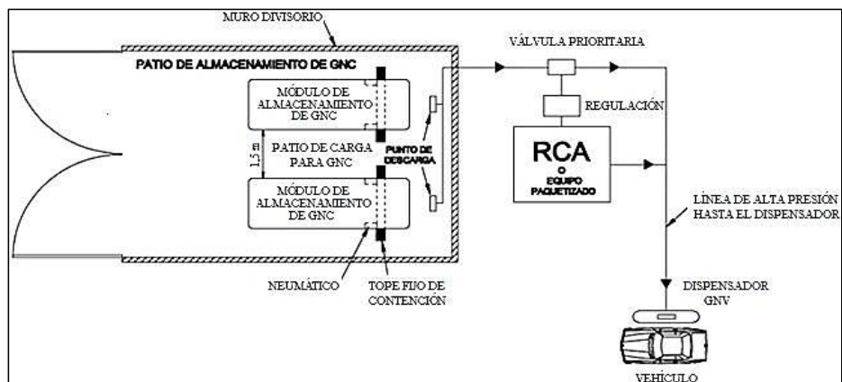
Figura 2A - Esquema referencial de una estación de descarga de GNC que descarga a una estación de GNV con pared divisoria 4TRF
