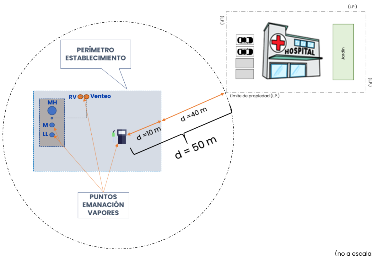
Figura 1: Representación gráfica de verificación de distancia mínima de seguridad desde centros afluencia al público
