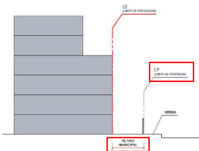
Figura 2: Representación gráfica de retiro municipal de establecimiento (Tomado de NORMA TÉCNICA G.040, DEFINICIONES DEL REGLAMENTO NACIONAL DE EDIFICACIONES, aprobado por RM N° 029-2021-VIVIENDA)
