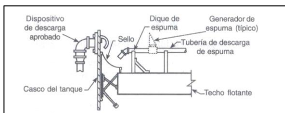
Gráfico 7.- Modelo de aplicación de espuma en superficie en tanque de techo flotante.
