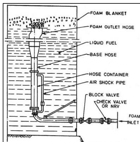
Gráfico 9.- Diagrama de Inyección de espuma semi-bajo superficie
