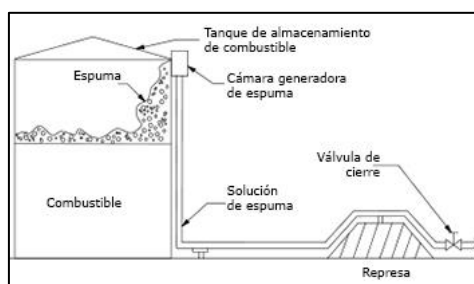
Gráfico 6.- Diagrama de aplicación de espuma en superficie en tanque de techo fijo.
