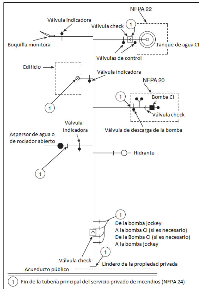
Gráfico 5. Tubería principal típica de un sistema de protección contra incendios
