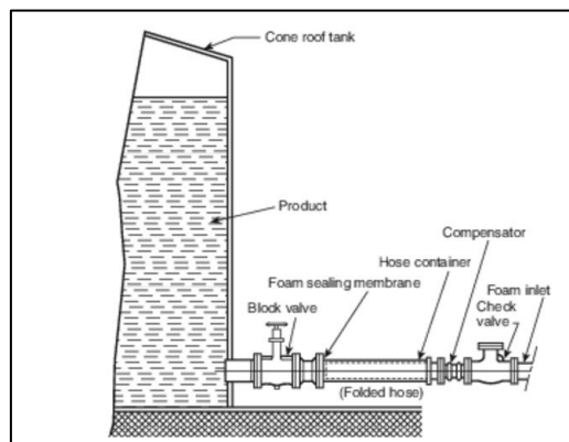
Gráfico 8.- Diagrama de Inyección de espuma bajo superficie
