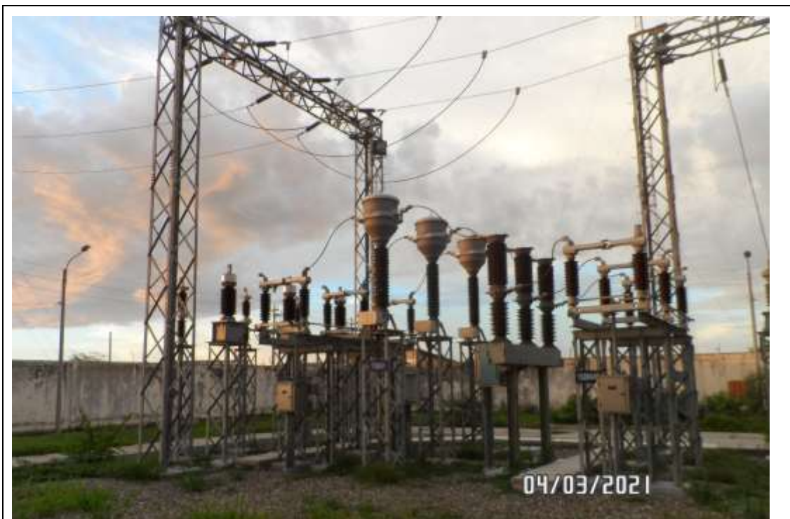
Foto 17. SET ZARUMILLA. Celda de línea 60 kV. Concluido el montaje electromecánico, falta el conexionado de equipos a barras. Obra paralizada por retiro del contratista.
