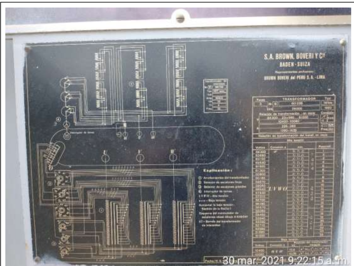
Foto 5. SET Industrial. Placa de características de transformador retirado definitivamente de operación.
