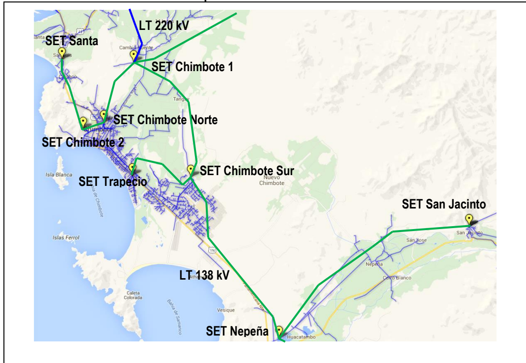
Gráfico N° 2.2: Principales Instalaciones del Área de Demanda 3
