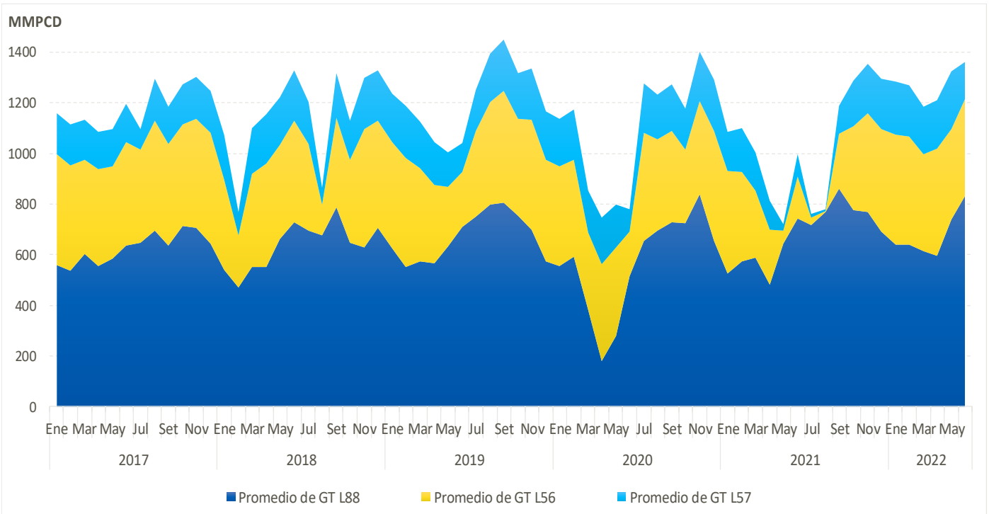
Gráfico 24. Gas Natural Transportado por Lotes (en MMPCD)
