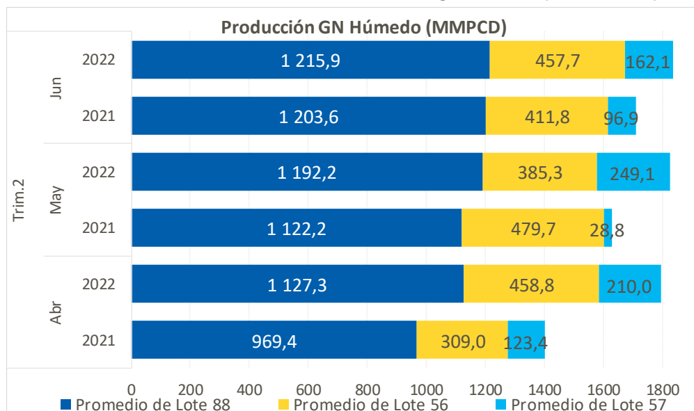
Gráfico 14. Comparación de Producción Promedio Mensual de Gas Natural Húmedo del Segundo Trimestre (2021-2 vs 2022-2), Principales Lotes (MMPCD)
