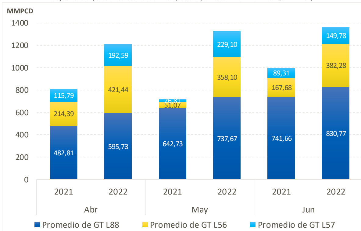
Gráfico 25. Comparación de Gas Natural Transportado por Lotes T2-2021 vs T2-2022(en MMPCD)
