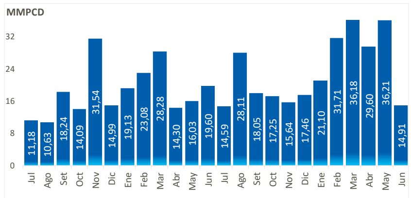
Gráfico 28. Volumen Transferido Entre Empresas Receptoras (en MMPCD)
