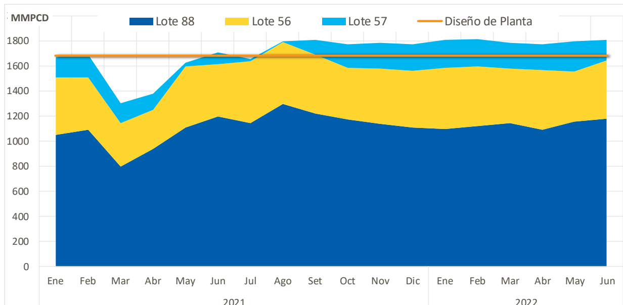
Gráfico 21 Gas Natural Procesado por Lotes y capacidad de Diseño de Planta (en MMPCD)
