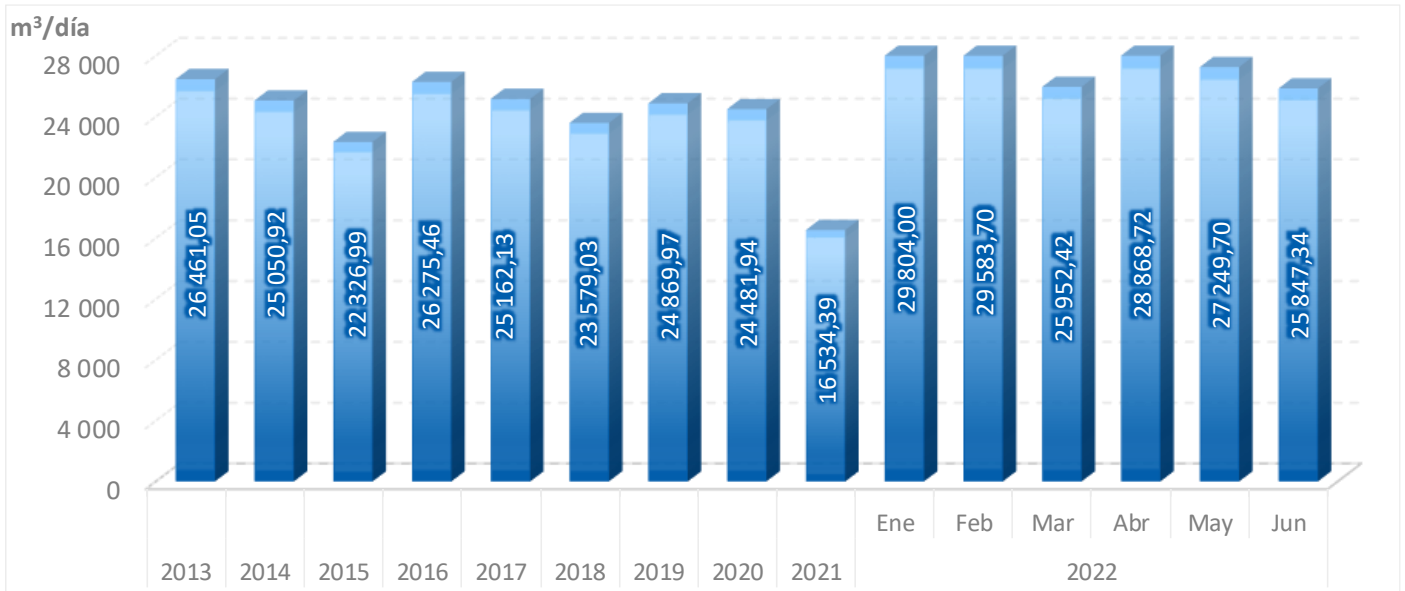
Gráfico 35. Gas Natural Licuefactado Producido en la Planta Melchorita, Promedio Mensual 2013-2022 (en m 3 /día)
