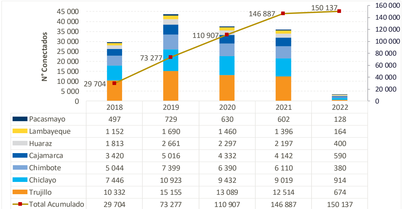
Gráfico 44. Primer Plan de Conexiones, Concesión Norte.
