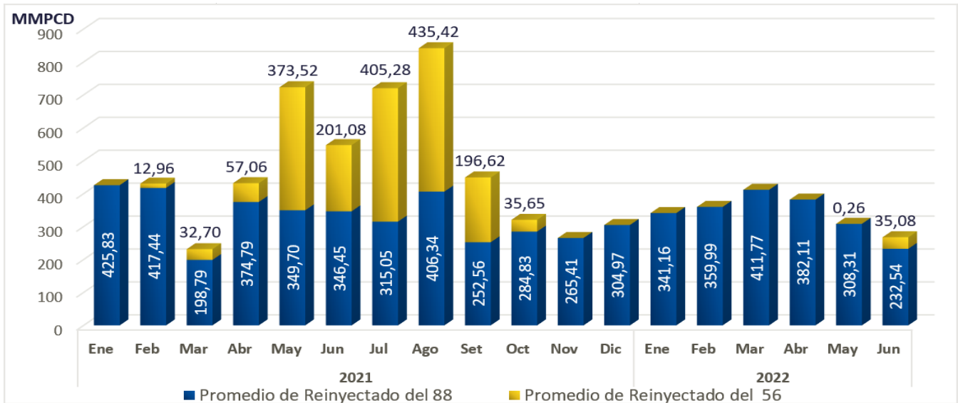
Gráfico 20. Reinyección de Gas Natural por Lotes (en MMPCD)
