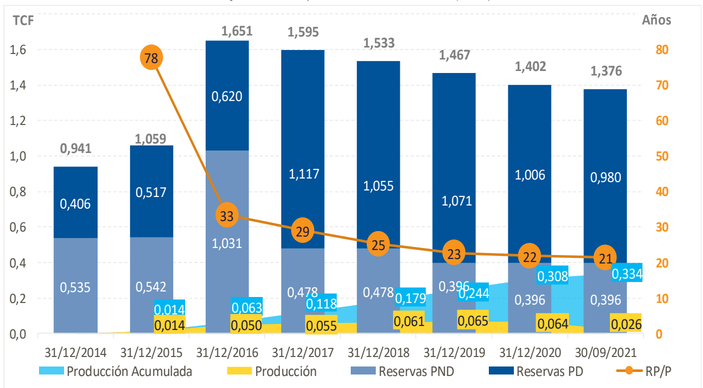
Gráfico 40. Reservas y Producción Acumulada. Lote 57 (en TCF)
