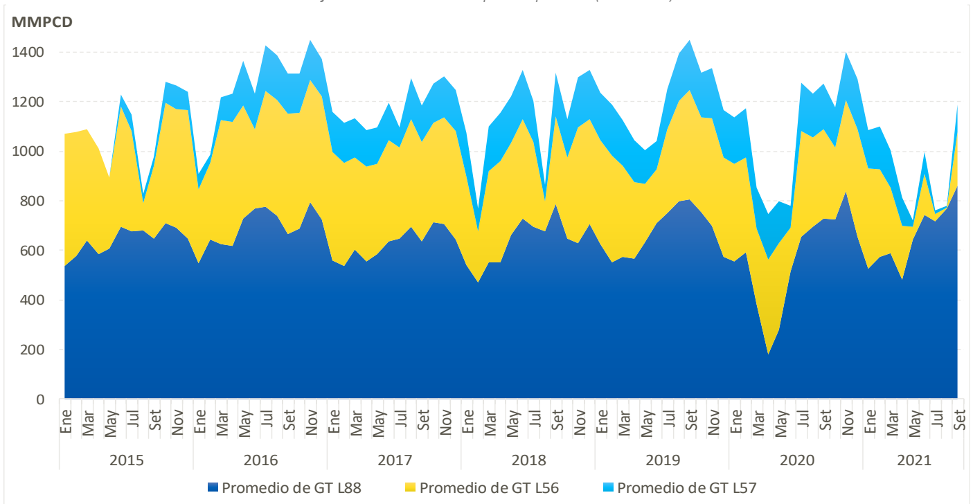
Gráfico 22.. Gas Natural Transportado por Lotes (en MMPCD)
