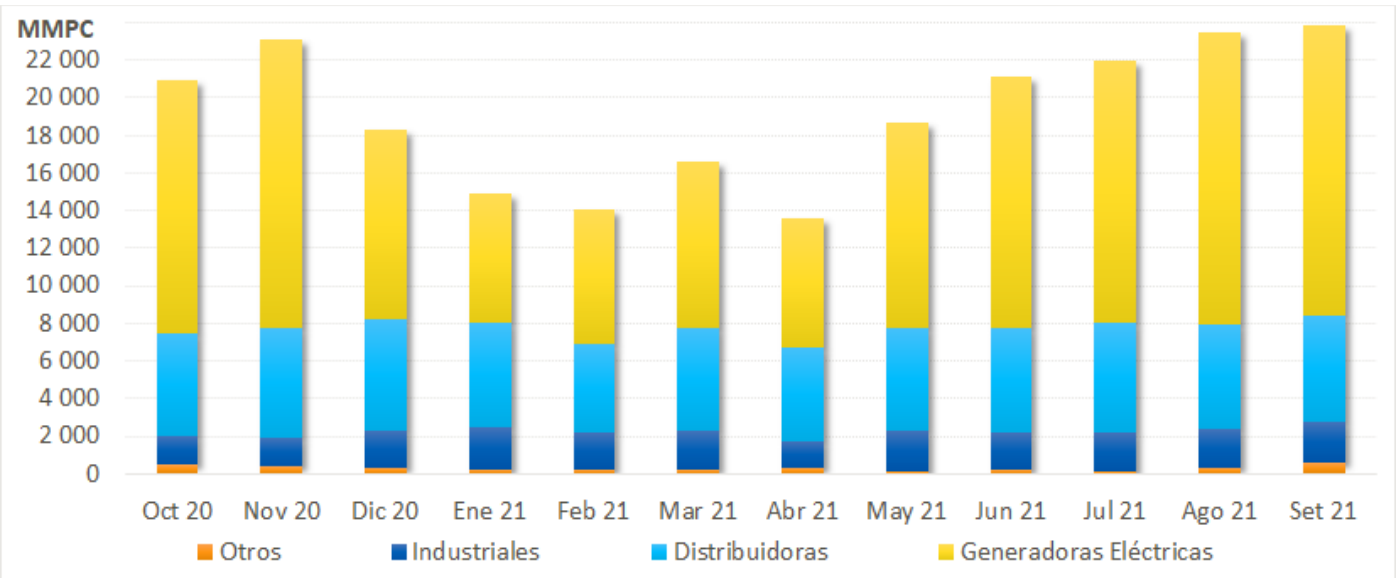
Gráfico 16. Ventas Mensuales de Pluspetrol al T3-2021, Lote 88 (en MMPC)
