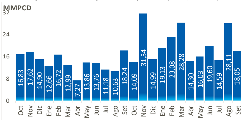
Gráfico 26. Volumen Transferido Entre Empresas Receptoras (en MMPCD)
