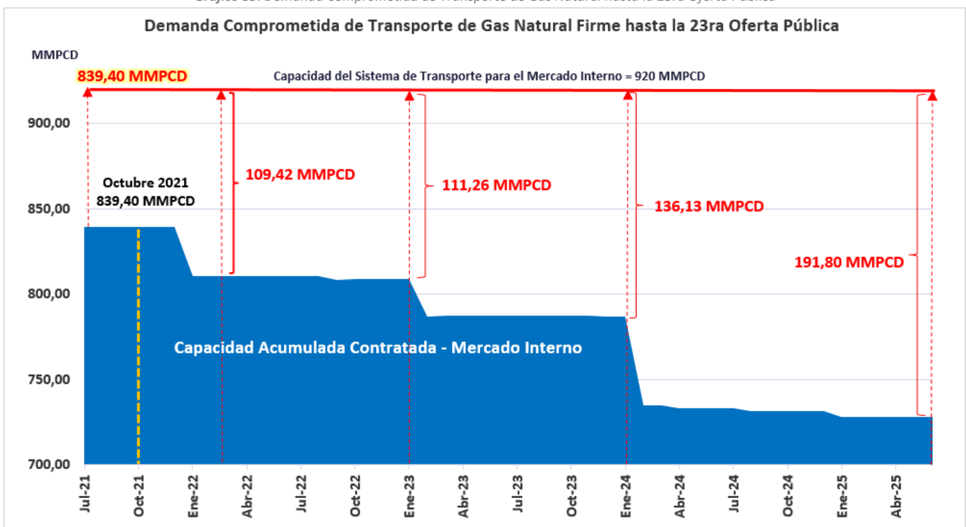
Gráfico 55. Demanda Comprometida de Transporte de Gas Natural hasta la 23ra Oferta Pública
