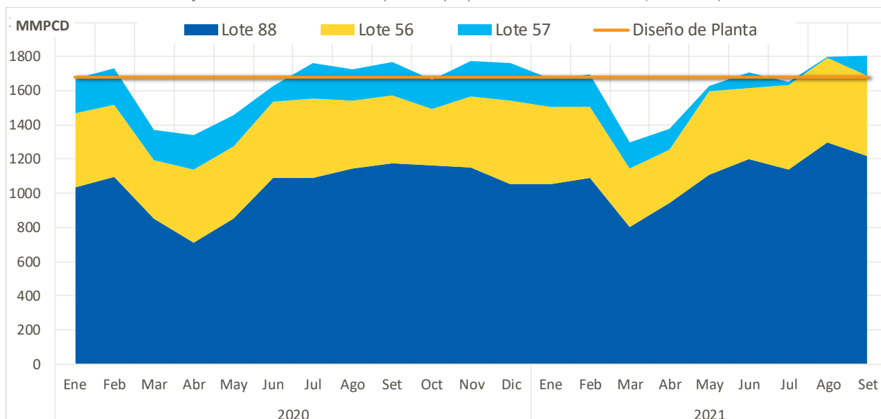
Gráfico 19. Gas Natural Procesado por Lotes y capacidad de Diseño de Planta (en MMPCD)
