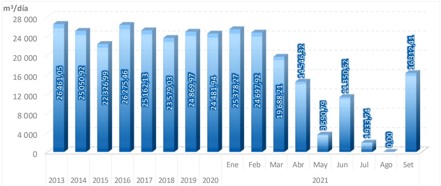
Gráfico 33. Gas Natural Licuefactado Producido en la Planta Melchorita, Promedio Mensual 2013-2021 (en MMPCD)
