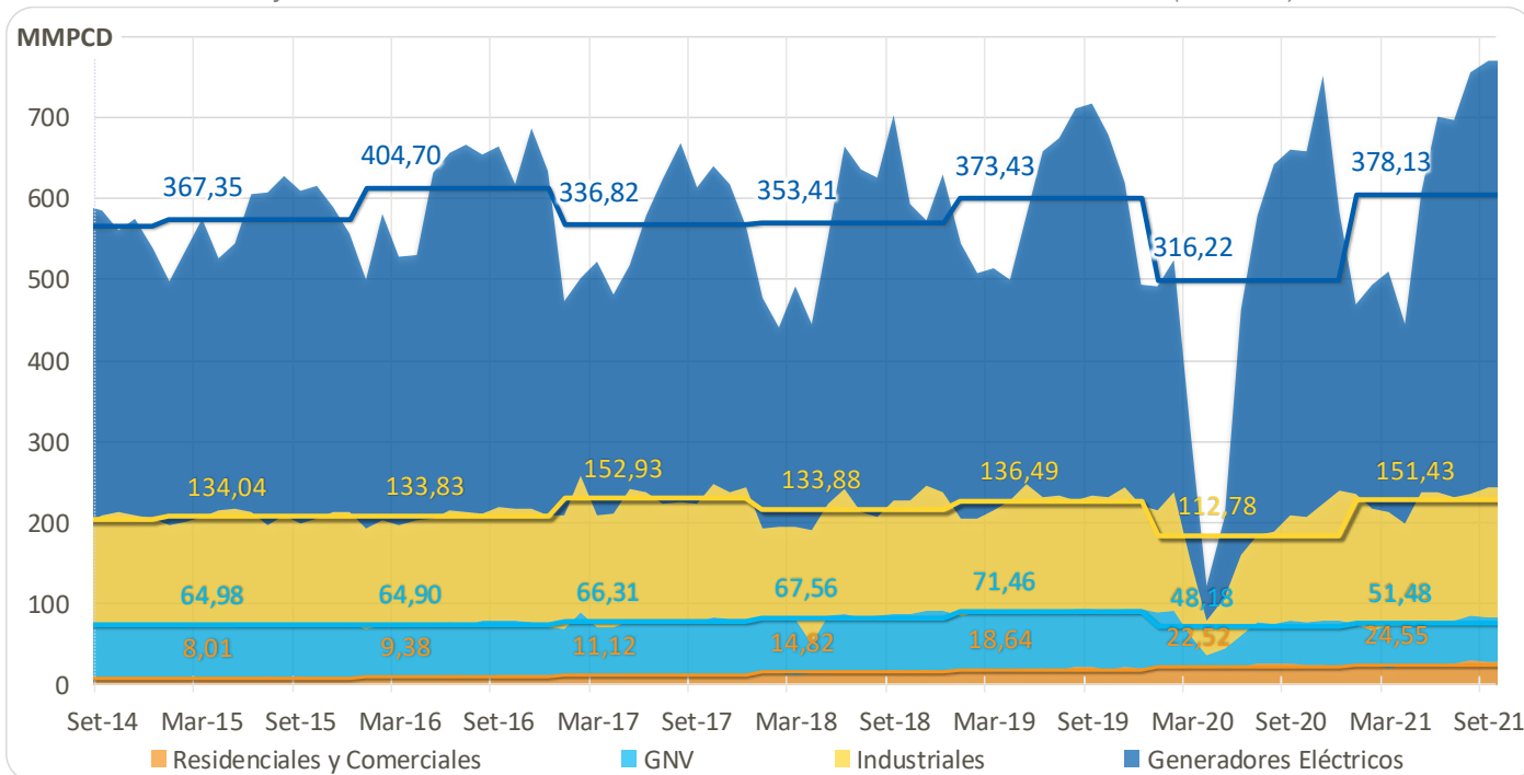
Gráfico 29. Consumo Promedio Mensual del Mercado Interno de Gas Natural de Camisea – 2021 (en MMPCD)
