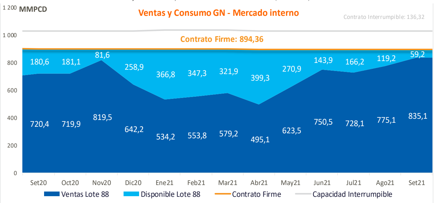
Gráfico 17. Ventas y Consumo Mensual de Gas Natural (en MMPCD)
