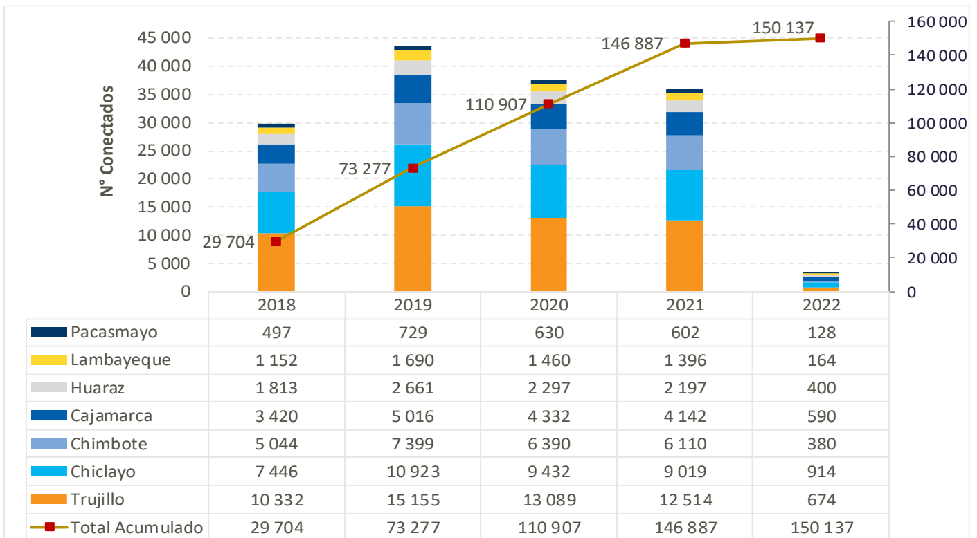
Gráfico 47. Primer Plan de Conexiones, Concesión Norte.
