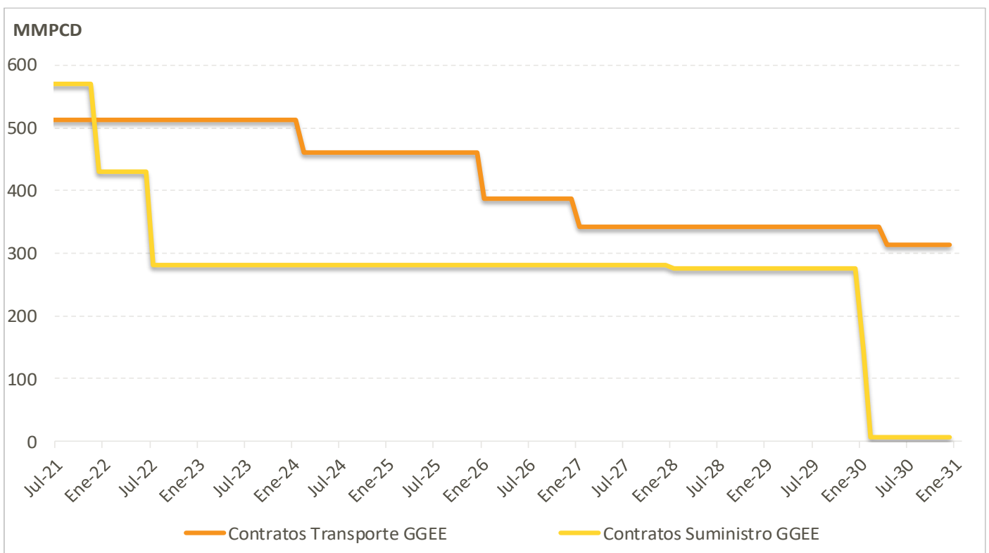
Gráfico 54. Contratos de Suministro vs. Contratos de Transporte. (en MMPCD)
