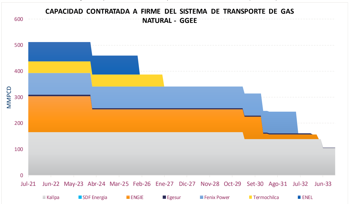
Gráfico 52. Capacidad Contratada de Transporte de Gas. Generadores Eléctricos (en MMPCD)
