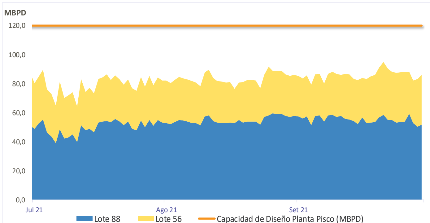
Gráfico 20. Líquidos de Gas Natural Procesados por Lote y capacidad de Diseño de Planta Pisco (en MBPD)
