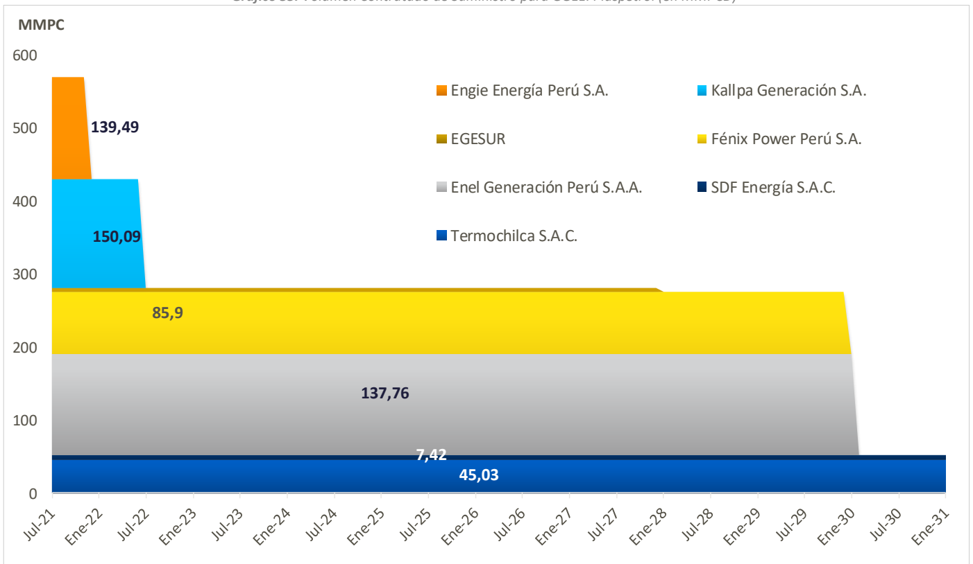
Gráfico 53. Volumen Contratado de Suministro para GGEE. Pluspetrol (en MMPCD)
