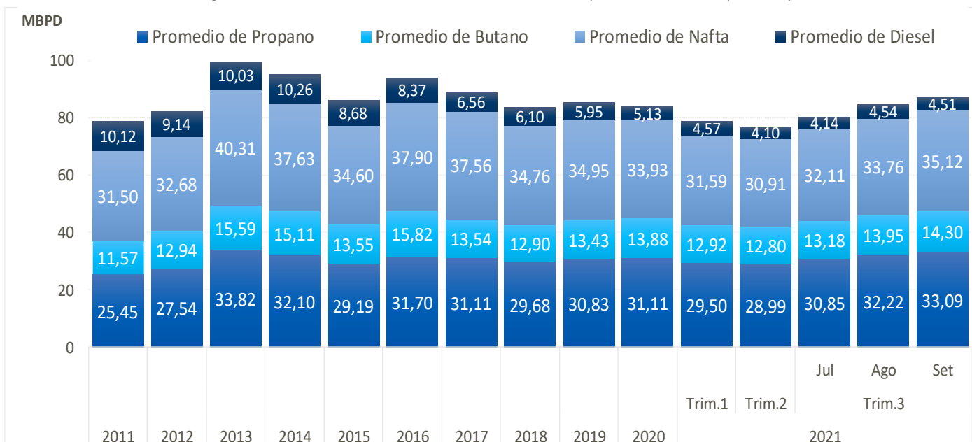
Gráfico 21. Productos Finales Obtenidos del Procesamiento de Líquidos de Gas Natural (en MBPD)
