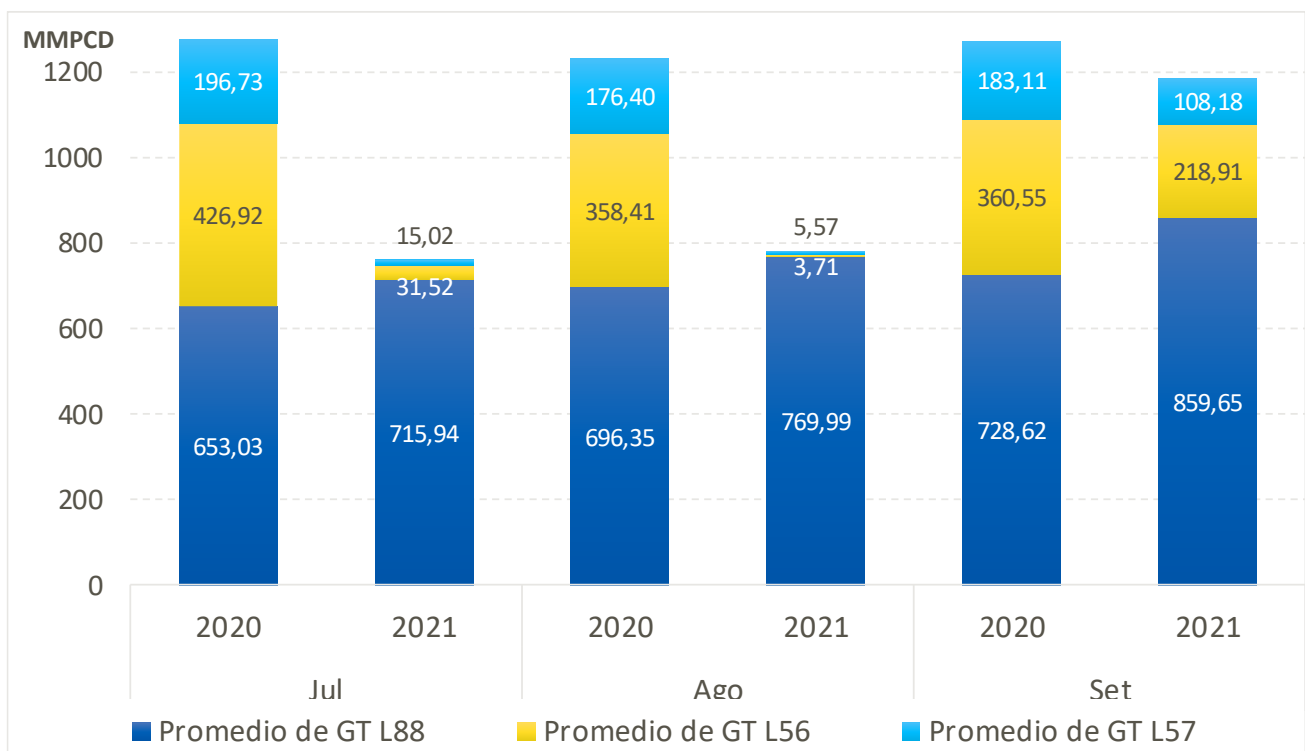
Gráfico 23.. Comparación de Gas Natural Transportado por Lotes T3-2020 vs T3-2021(en MMPCD)
