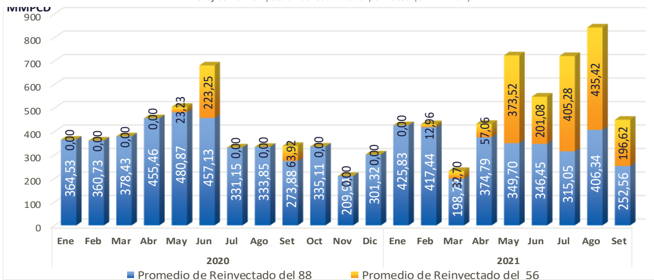
Gráfico 18. Reinyección de Gas Natural por Lotes (en MMPCD)
