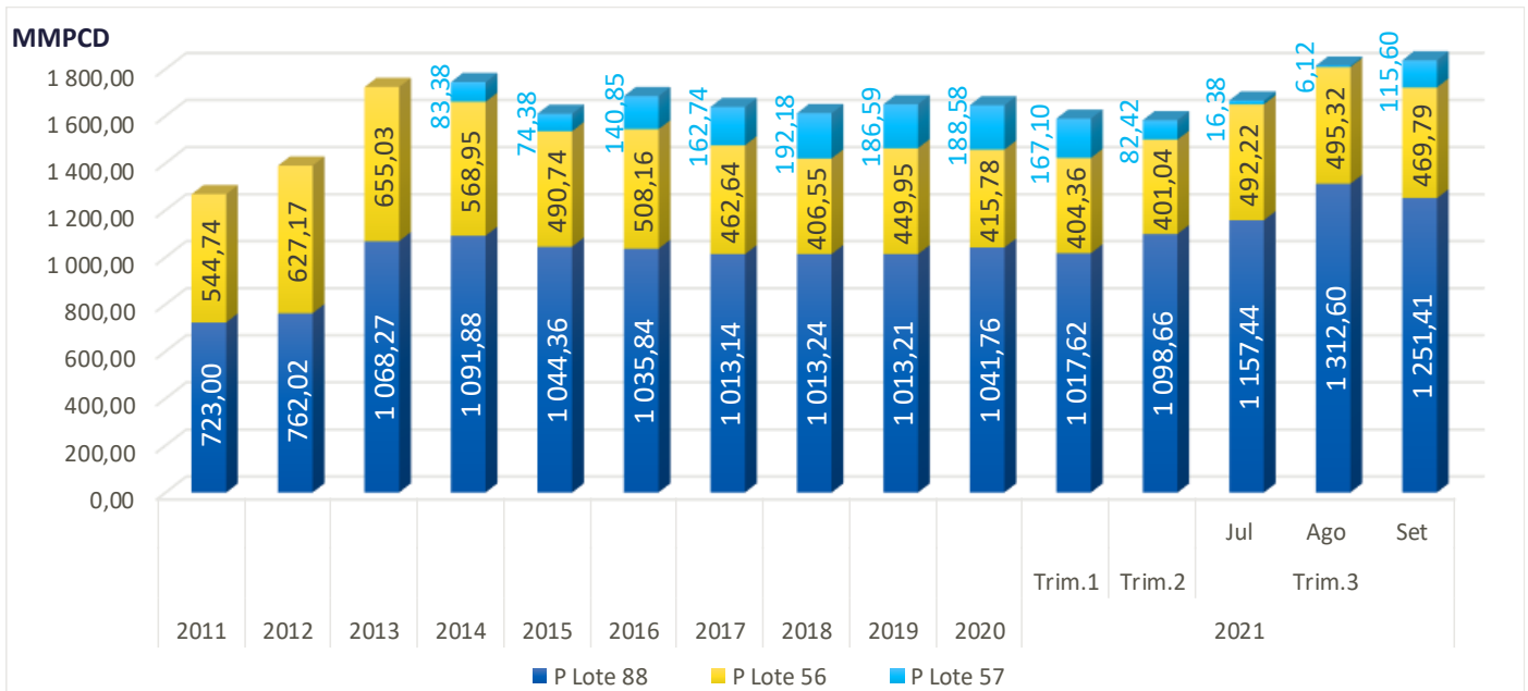
Gráfico 11. Producción Promedio Mensual de Gas Natural Húmedo al 2021, Principales Lotes (en MMPCD)
