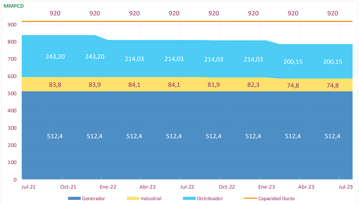
Gráfico 51. Capacidad Contratada de Transporte Firme. TgP (en MMPCD)
