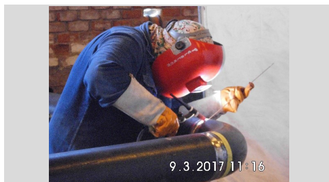
Soldadura de tubería en el taller de Mecor, proyecto City Gate, distrito de San Vicente de Cañete y provincia de Cañete.
