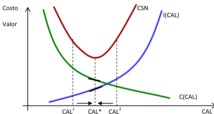
Gráfico N° 1 Costos y beneficios de la provisión de calidad
